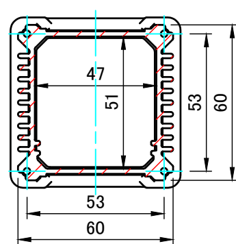
A-A ( 1 : 2 )
